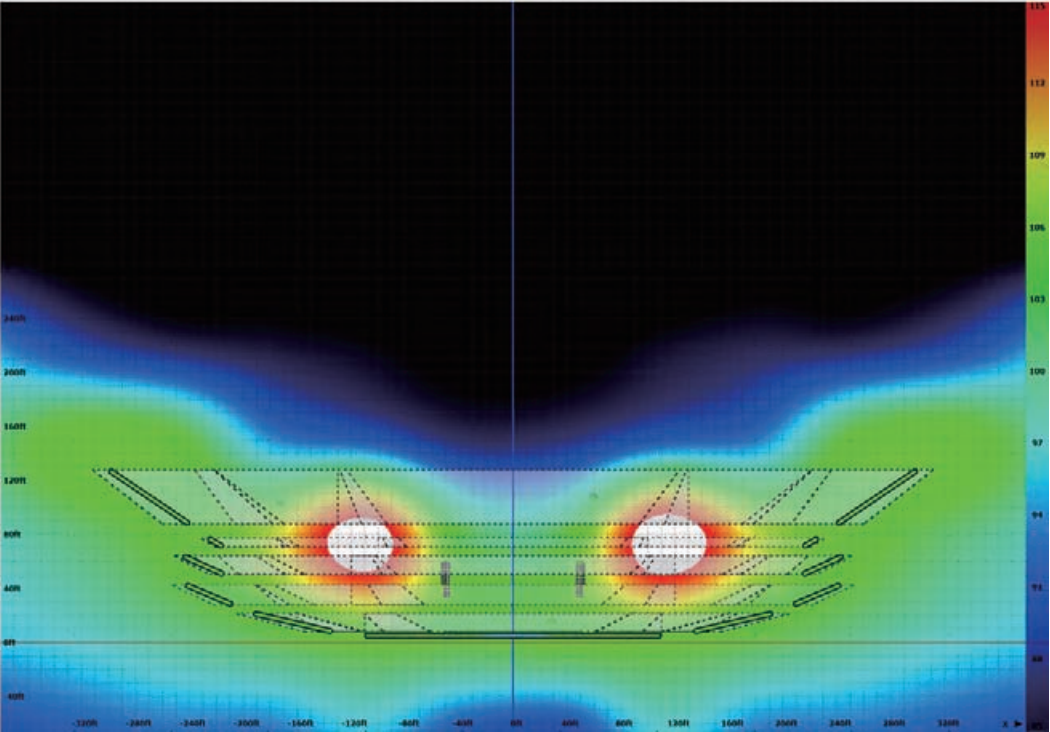
场地剖视图
