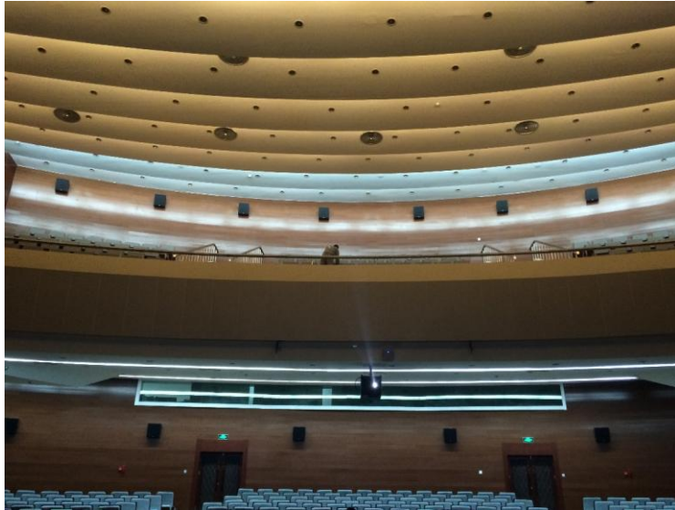
大会议厅安装了 22 只 EAW CR72z 环绕声音箱，营造极强的浸入感
