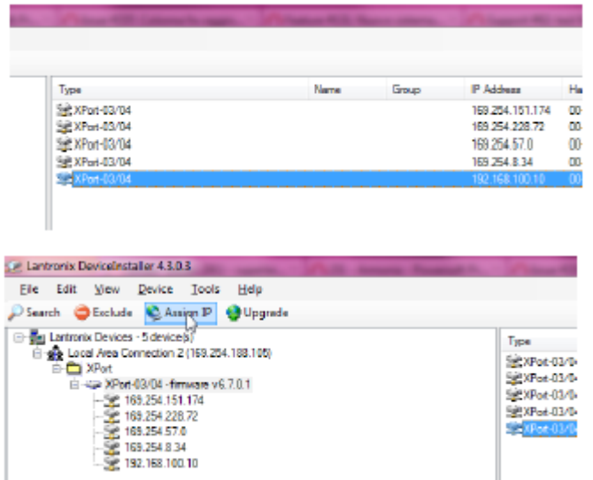
图 2: 在右面板选择设备，点击分配 IP。
